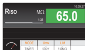
Misura di resistenza di isolamento
