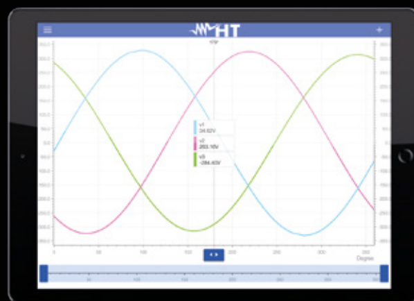
Forme d'onda di tensione e corrente.
