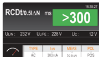
Test su differenziali RCD
