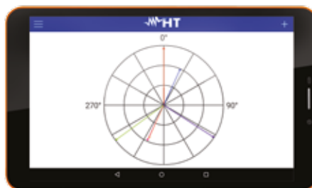
Esempio di visualizzazione Fasori in tempo reale
