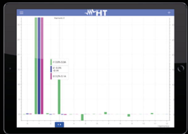
Armoniche di corrente e tensione.
