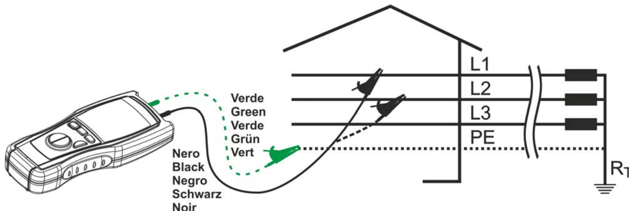
Fig. 7 : Connexion des bornes de l'instrument dans l'essai ⚠
