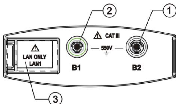
Fig. 2 : Description des entrée de l'instrument
