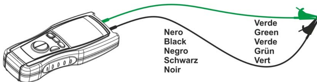
Fig. 6 : Connexion des bornes pendant la procédure de calibration
