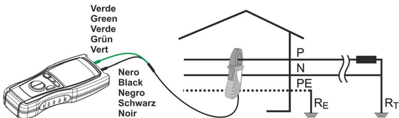
Fig. 4 : Connexion des bornes de l'instrument dans l'essai A \approx HZ
