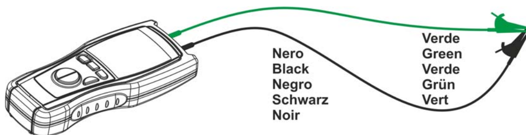
Fig. 10 : Connexion des bornes pendant la procédure de calibration
