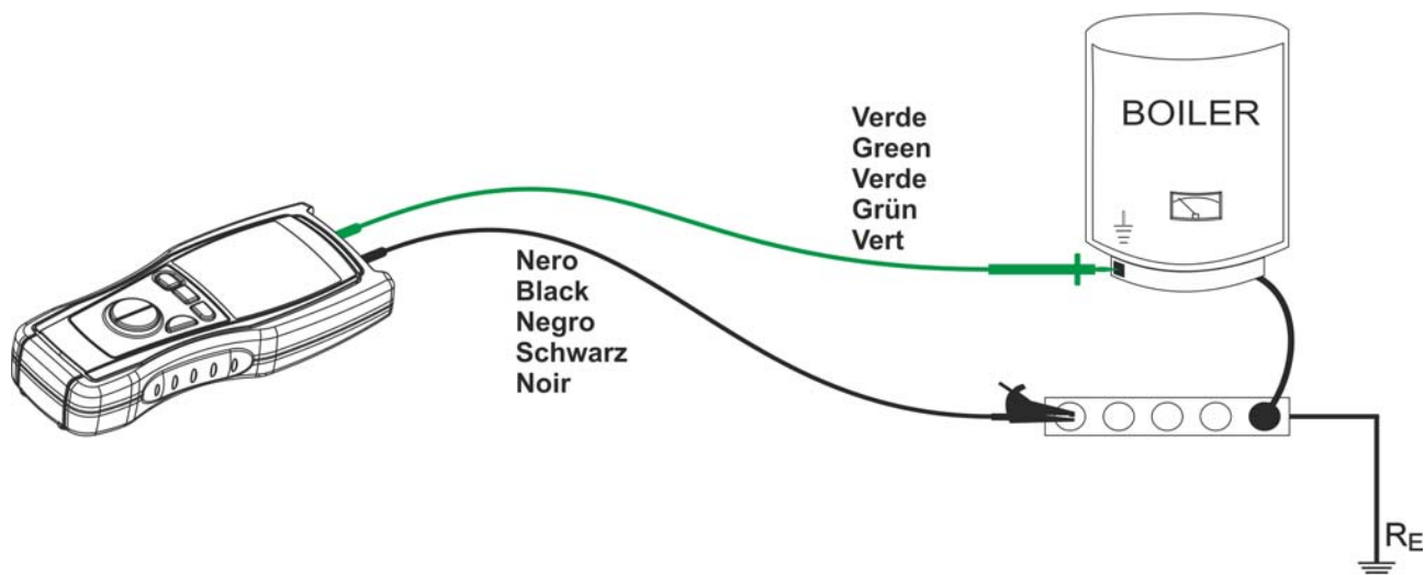
Fig. 9 : Connexion des bornes de l'instrument dans l'essai \Omega 0.2A
