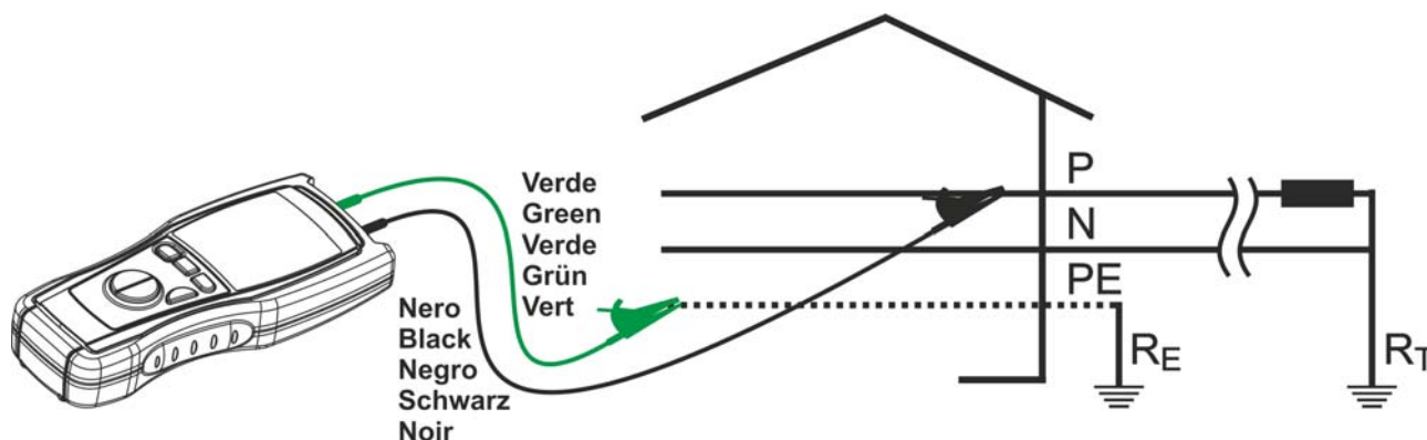
Fig. 3 : Connexion des bornes de l'instrument pour mesures V \approx Hz
