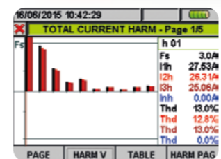
Visualizzazione delle armoniche di corrente in real time
