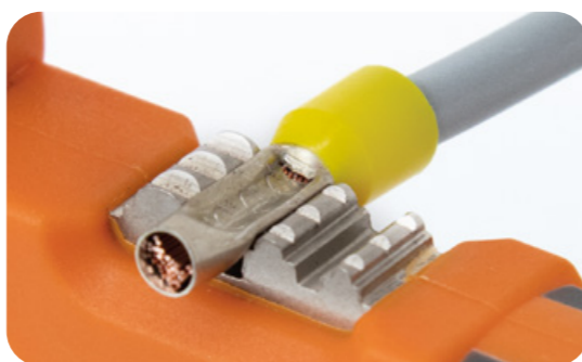
Puntalino da 4mm 2 crimpato con F40
