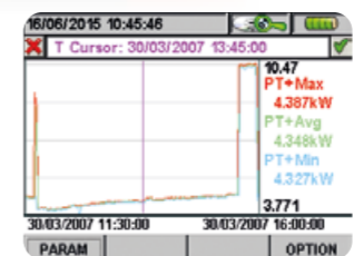
Visualizzazione grafico della potenza registrata
