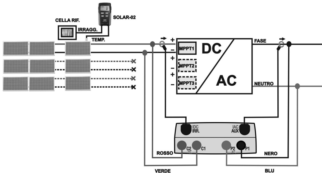
Fig. 4: Collegamento dello strumento per collaudo su impianto FV Monofase
