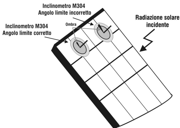
Fig. 7b: Posizionamento inclinometro M304
