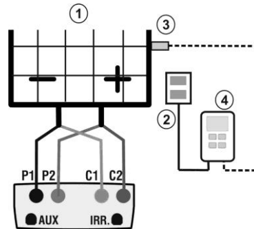
Fig. 15: Connessioni dello strumento per prove IVCK con mis. di Irragg/Temp tramite SOLAR-02
