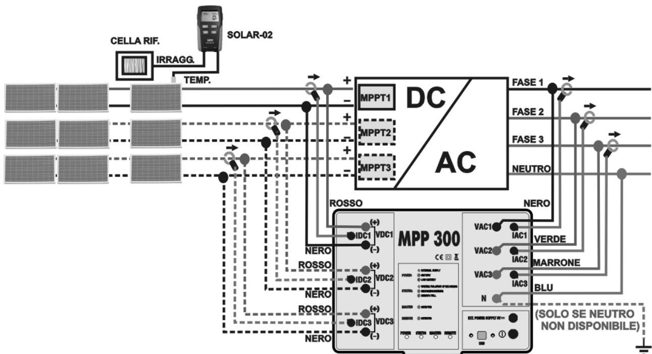
Fig. 6: Collegamento dell'MPP300 per collaudo di un impianto FV Trifase
