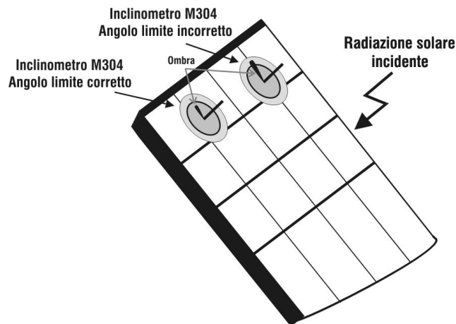
Fig. 8: Posizionamento inclinometro M304
