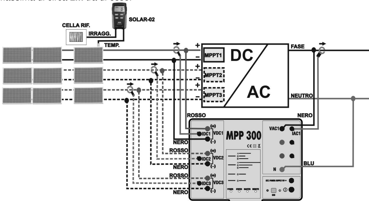
Fig. 5: Collegamento dell'MPP300 per collaudo di un impianto FV Monofase
