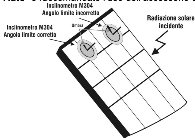
Fig. 10: Posizionamento inclinometro M304
