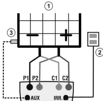
Fig. 14: Connessioni dello strumento per prove IVCK con mis. Diretta di Irragg/Temp
