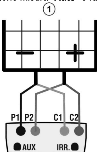
Fig. 13: Coll. strumento al modulo/stringa FV per prove IVCK senza misura mis. Irragg.
