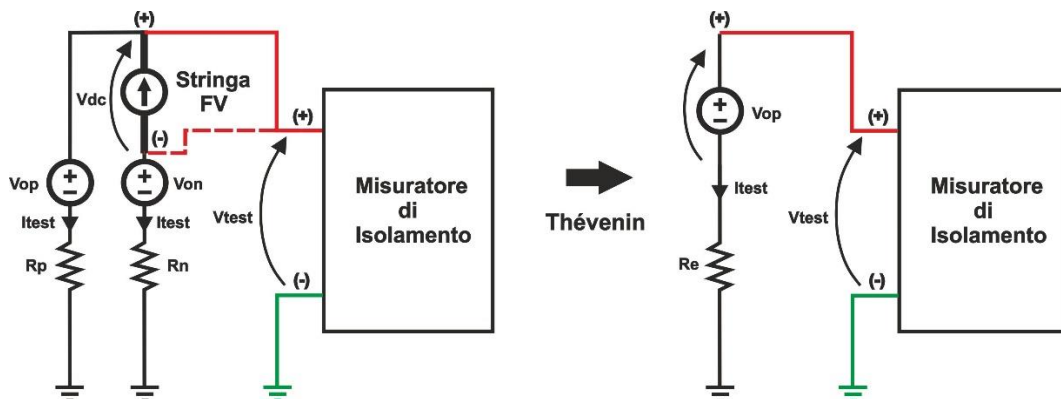
Fig. 17: Schema e circuito equivalente del Metodo 1
