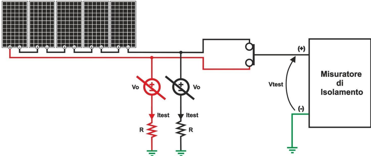
Fig. 18: Schema e circuito equivalente del Metodo 2
