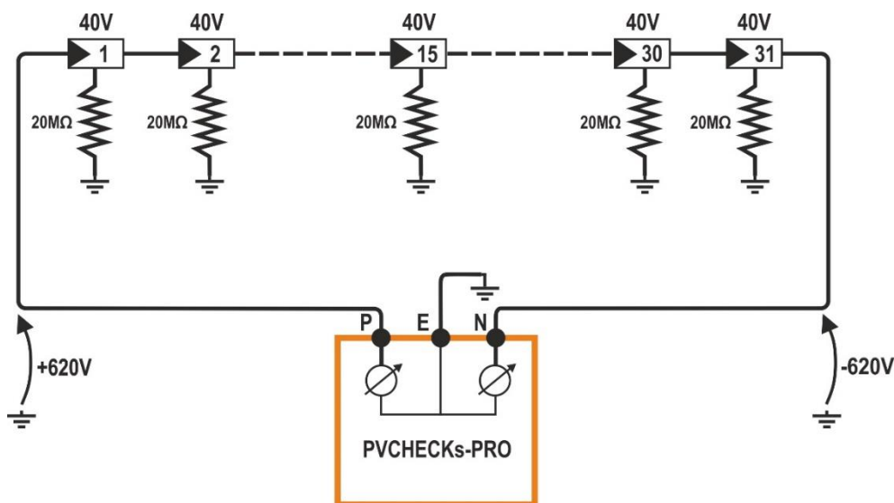
Fig. 16: Esempio di utilizzo della funzione GFL
