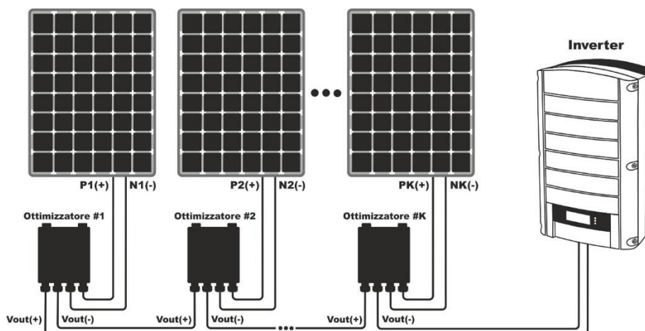
Fig. 19: Collegamento di una stringa FV con presenza di ottimizzatori di potenza
