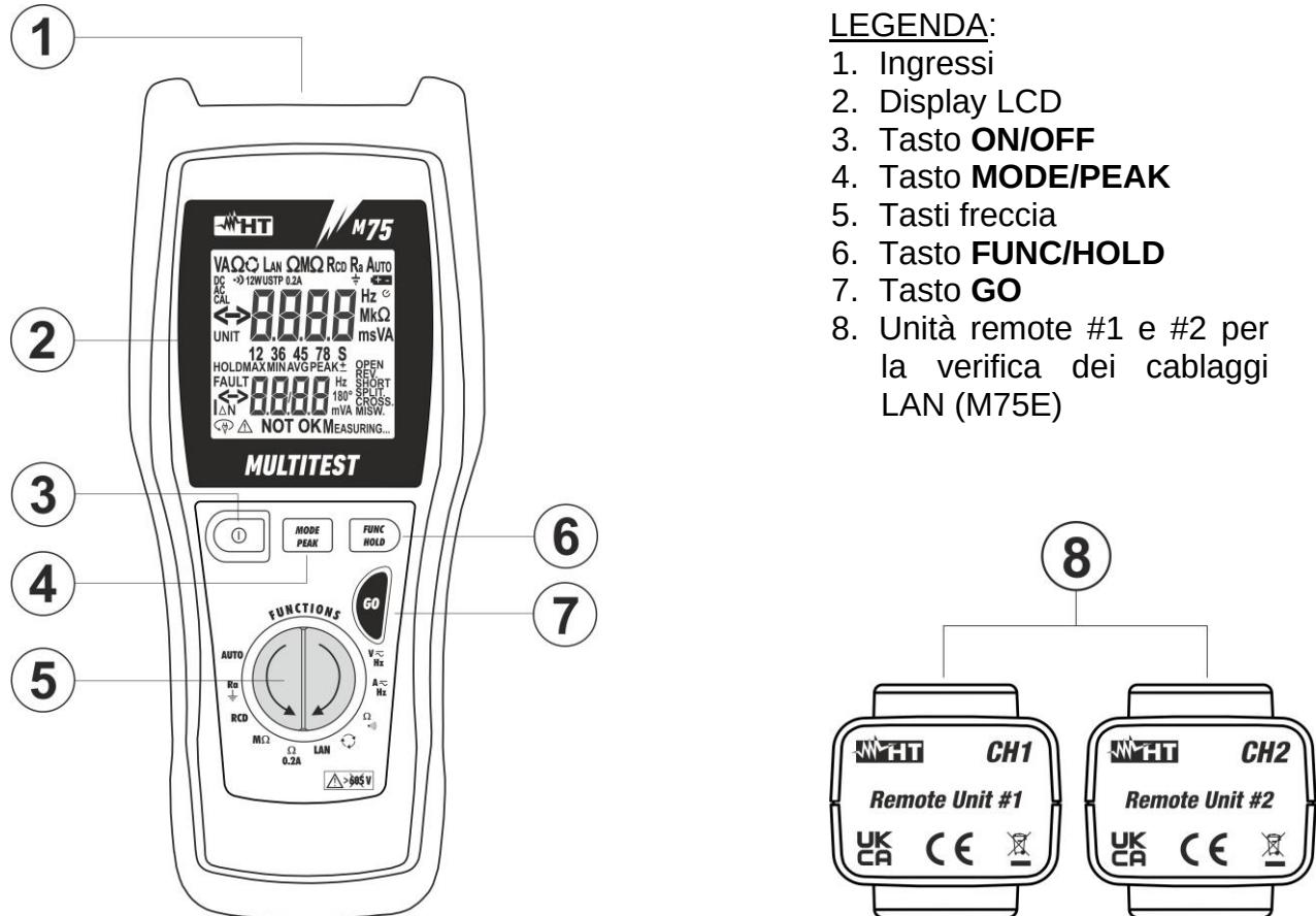
Fig. 1: Descrizione dello strumento
