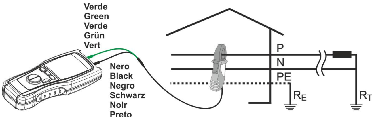
Fig. 4: Connessione dei terminali dello strumento
