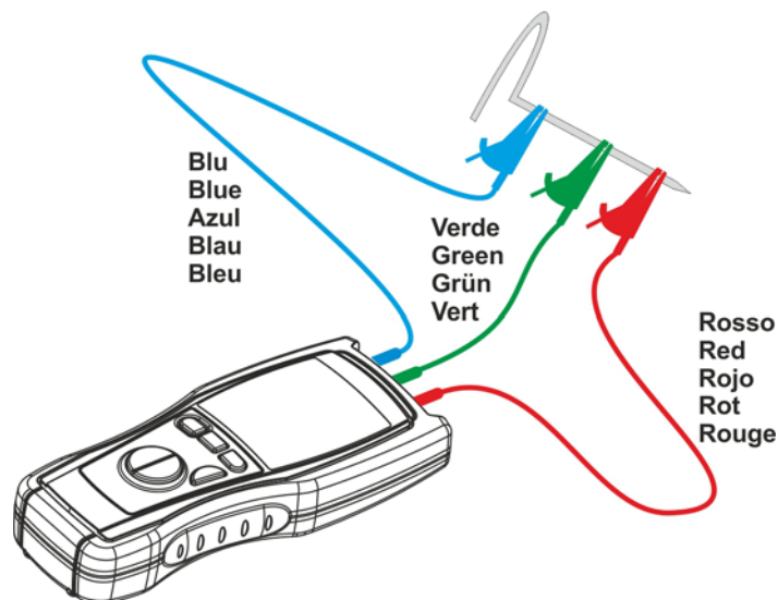
Fig. 5: Connessioni dello strumento per l'azzeramento dei cavi in modalità EARTH-3P
