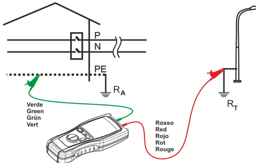
Fig. 3: Esempio di connessione dello strumento per la misura di Terra a 2 Punti
