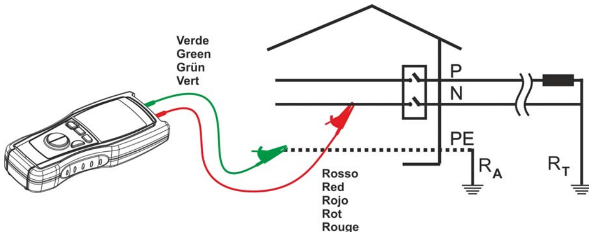
Fig. 4: Esempio di connessione dello strumento per la misura di Terra a 2 Punti (utilizzabile solo per sistemi TT).
