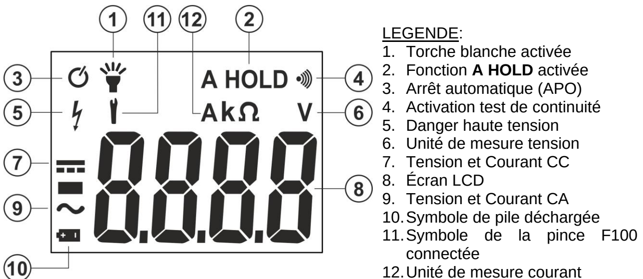
Fig. 2: Description des symboles de l'afficheur
