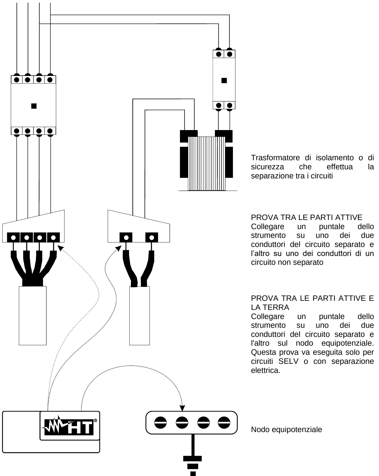
Fig. 44: Misure di separazione tra circuiti in un impianto
