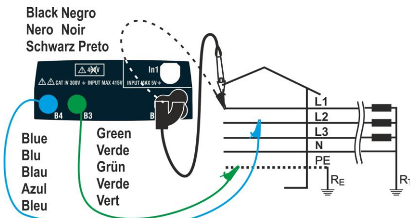
Fig. 28: Test L1-L2 per sistemi Trifase con cavi singoli e puntale remoto
