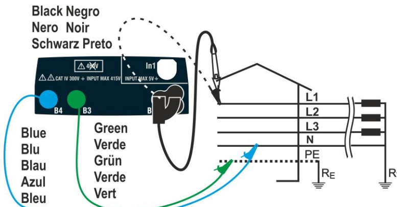
Fig. 27: Test L-N/L1-PE per sistemi Trifase con cavi singoli e puntale remoto
